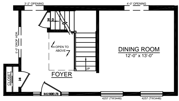
3BEDROOM OPEN SW OPTION
