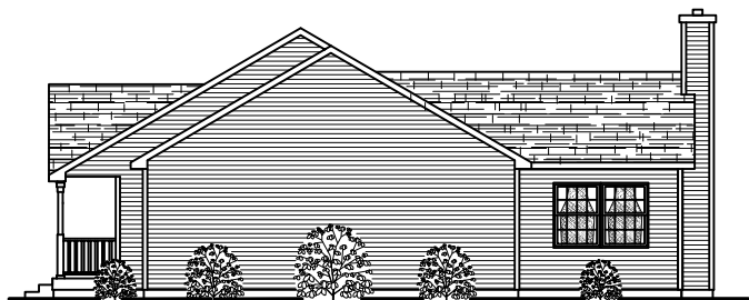
RIGHT ELEVATION
