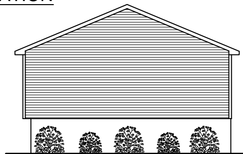
RIGHT ELEVATION
