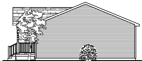
RIGHT ELEVATION
