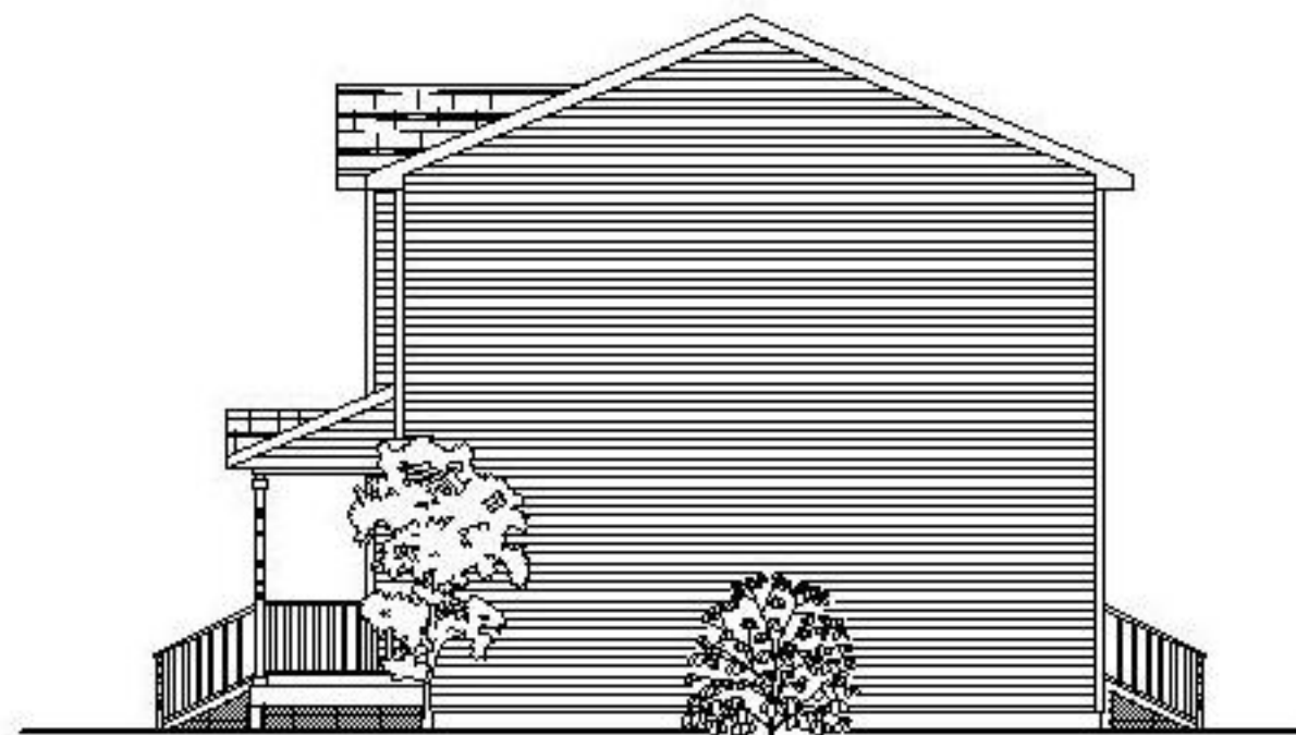
RIGHT ELEVATION
